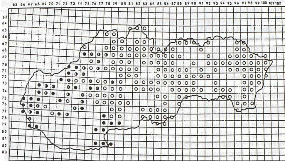
Mapa 10. ○ Pulmonaria obscura Dumort. ● Pulmonaria officinalis L. ⊙ spoločný výskyt oboch taxónov
